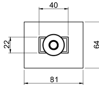
Foratura 40x22
